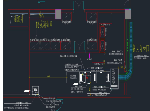
三楼布置图
